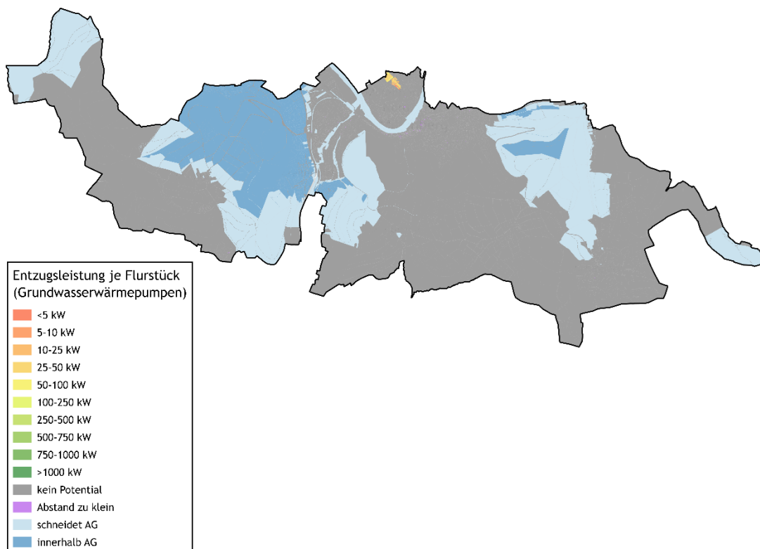
Abbildung 38: Entzugsleistung je Flurstück bei der Nutzung von Grundwasserwärmepumpen [11]
